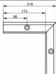
Verbinder – Bodenmontage Innenecke
