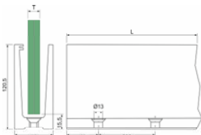
Bodenprofile – Bodenmontage
